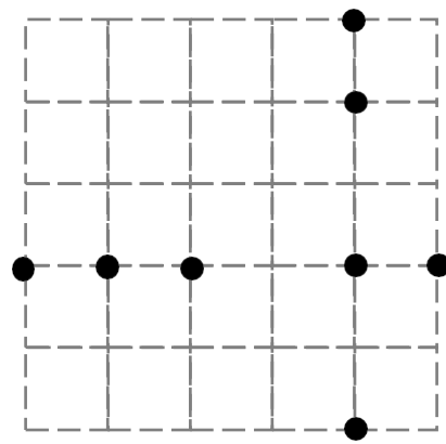
Trapezium
